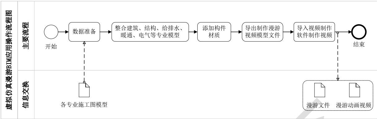
图33 虚拟仿真漫游 BIM 应用操作流程图
