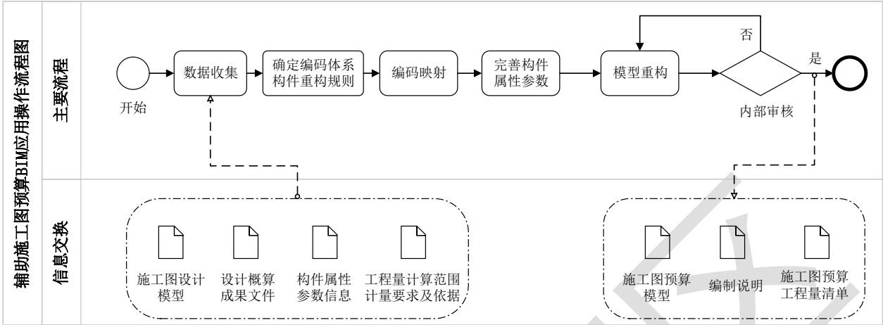
图37 辅助施工图预算 BIM 应用操作流程
