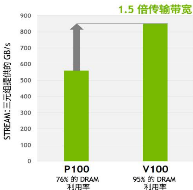
图 15. V100 上 HBM2 内存加速与 P100 的对比
