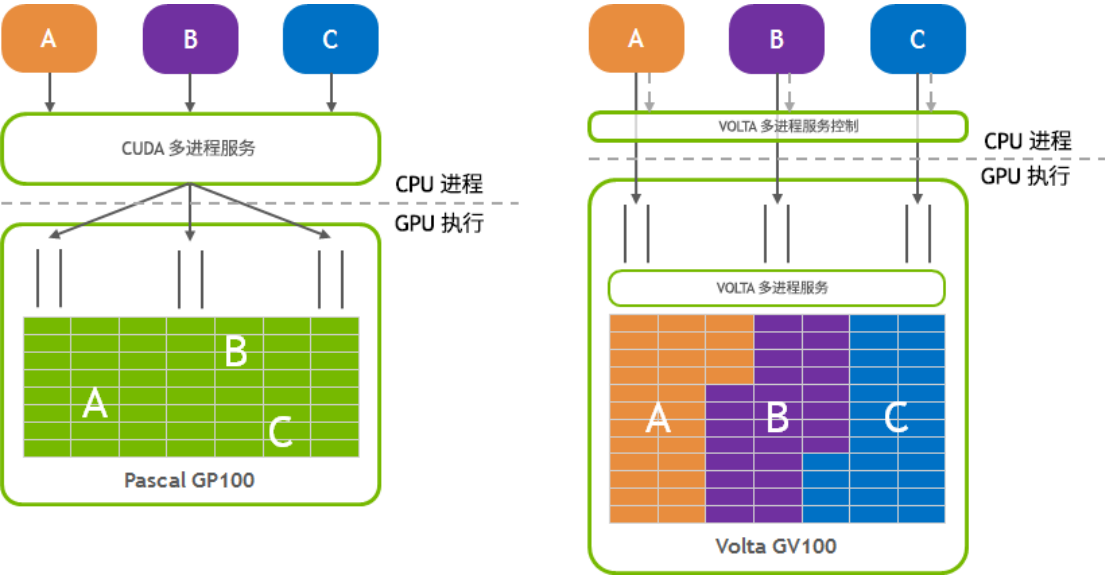
图 25. Pascal 中基于软件的 MPS 服务与 Volta 中硬件加速 MPS 服务的对比
