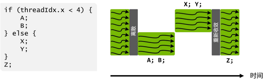
Pascal 和早期 NVIDIA GPU 的 SIMT 线程束执行模型中的线程调度。大写字母代表以程序伪代码编写的语句。线程束中离散的分支经过序列化，因此分支一侧的所有语句一起执行直至完成，然后另一侧的语句才会执行。执行 else 语句后，线程束的线程通常将重新收敛。
